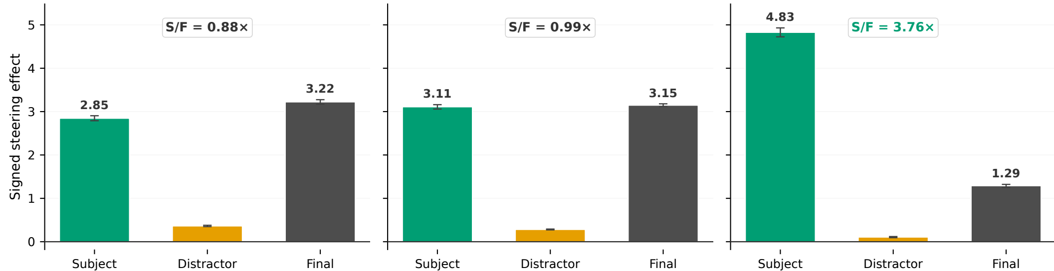
Phi-2
