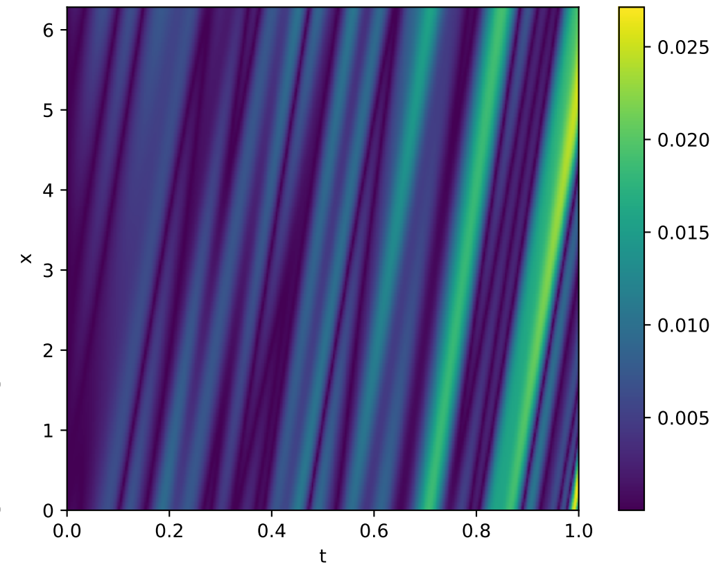
Absolute error
