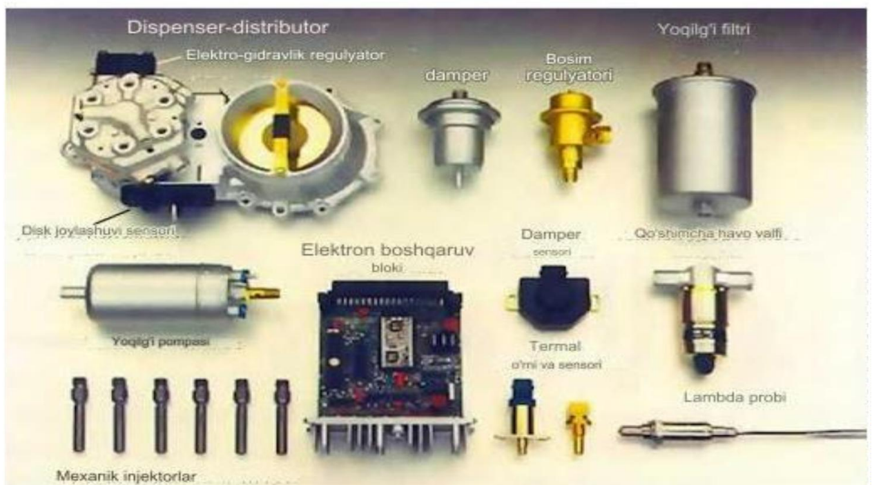
Yonilg‘i uzatish tizimi.
