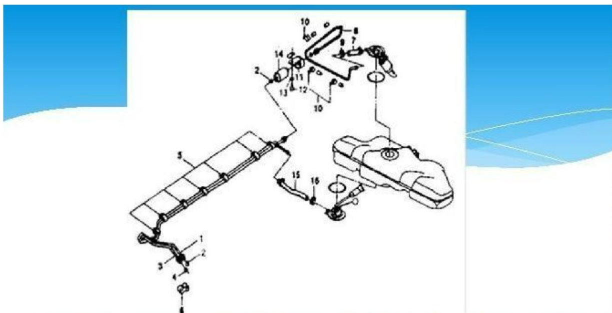
1-rasm. Nexia avtomobili dvigateling yonilg'ini purkash sistemasi sxemasi
