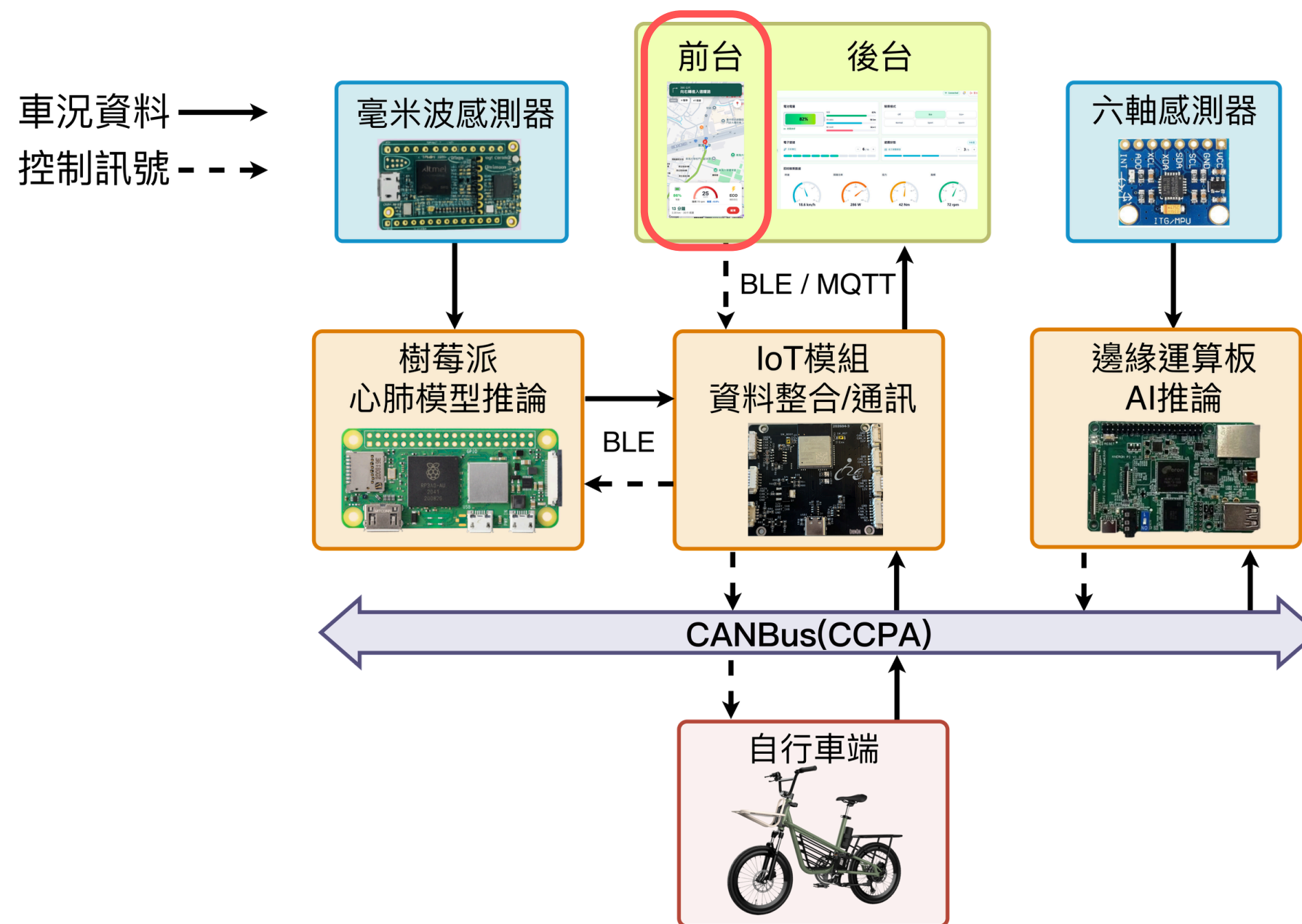
整車架構圖
