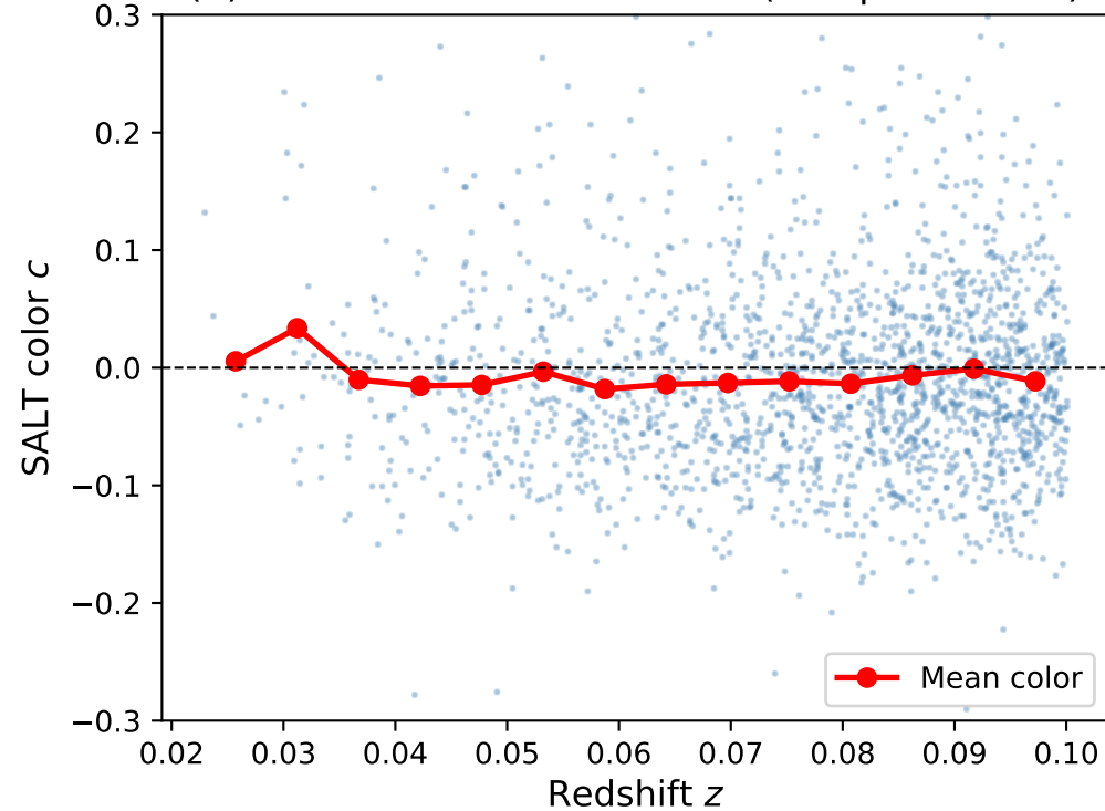
(d) Color--redshift correlation ( \tau depends on z )
