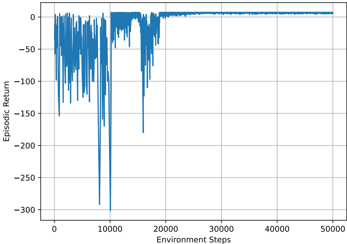
GWB Episodic Return
