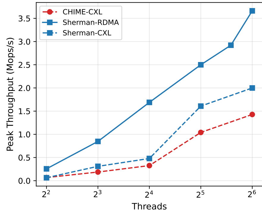
YCSB E
