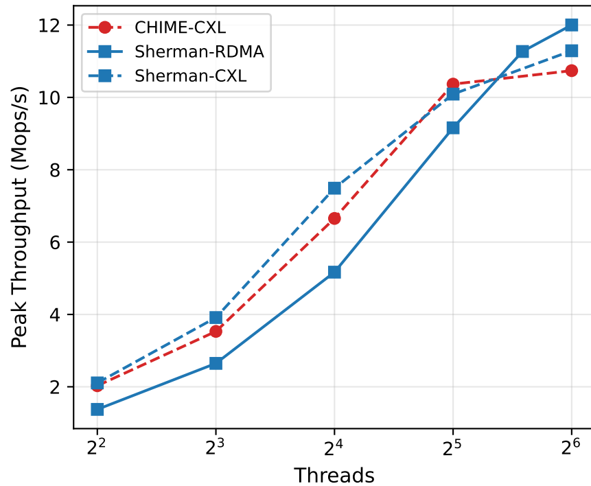
YCSB D
