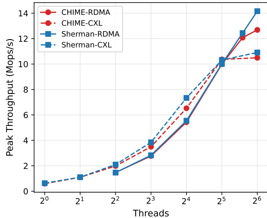
YCSB C
