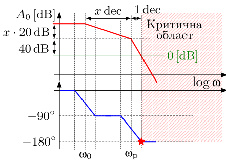
Слика 28.2: апроксимативне Бодјеове карактеристике, амплитудска и фазна.
