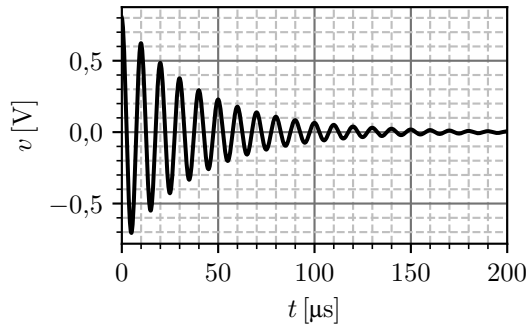
(б) Одскочни одзив у временском домену
