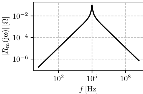
(а) Бодјева амплитудска карактеристика
