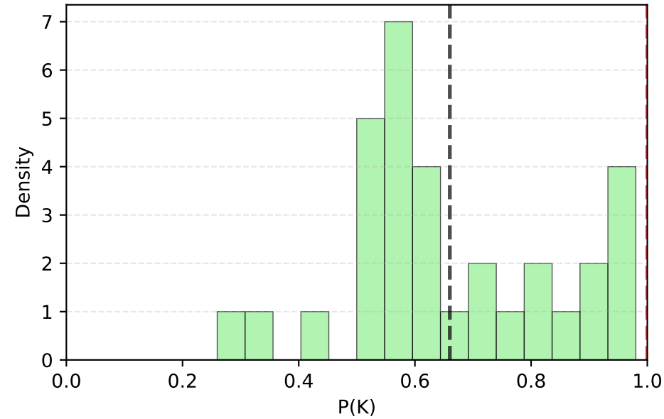
J(K vs R) - LSP \mu : 0.660 | Obj: 1.000 | n=32
