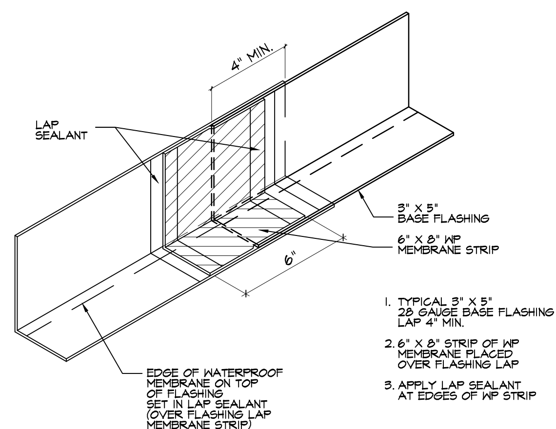
06 Flashing Lap SCALE: 3" = 1'-0"
