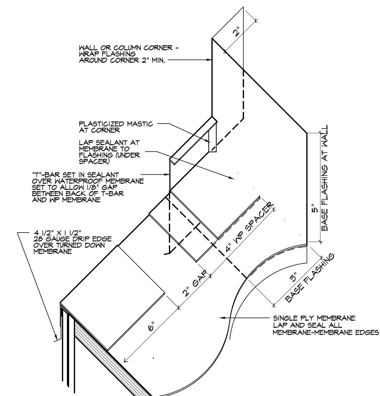
02 T Bar at Wall SCALE: 6" = 1'-0"
