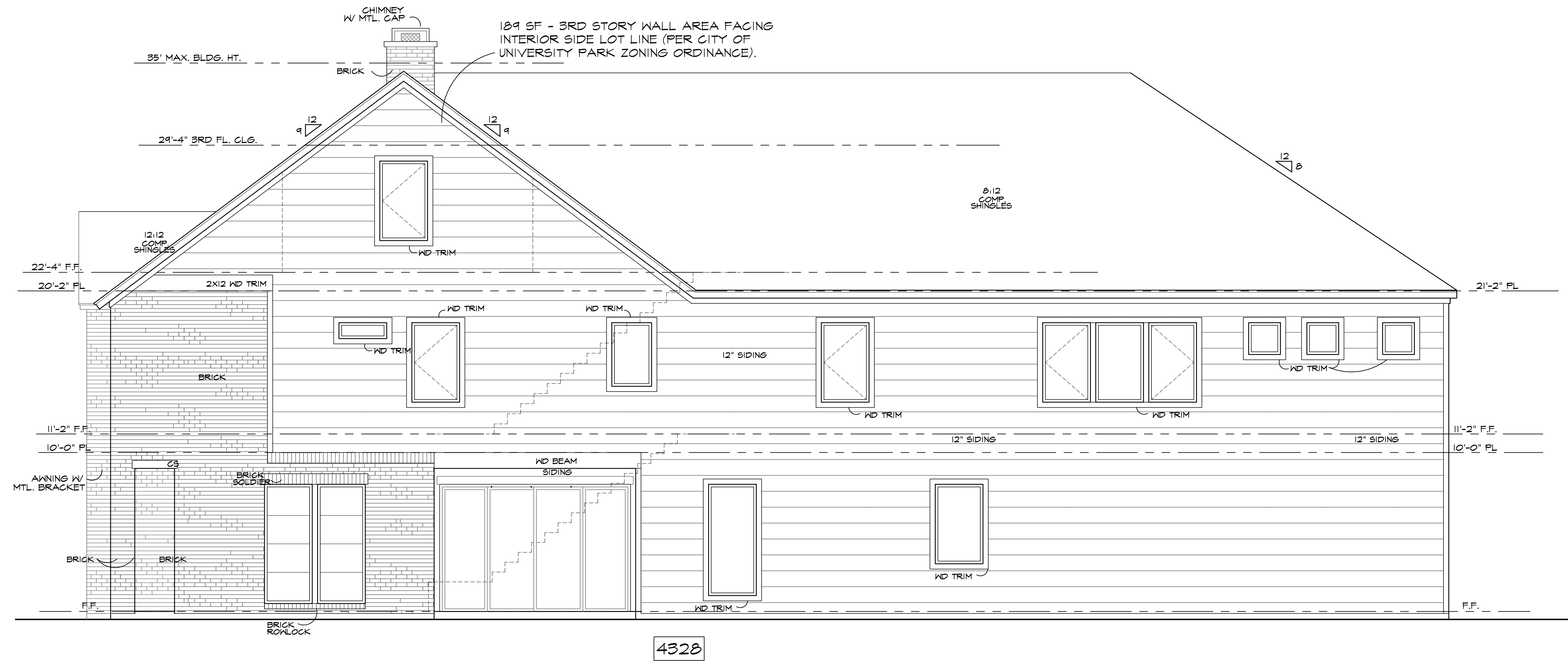
RIGHT ELEVATION
