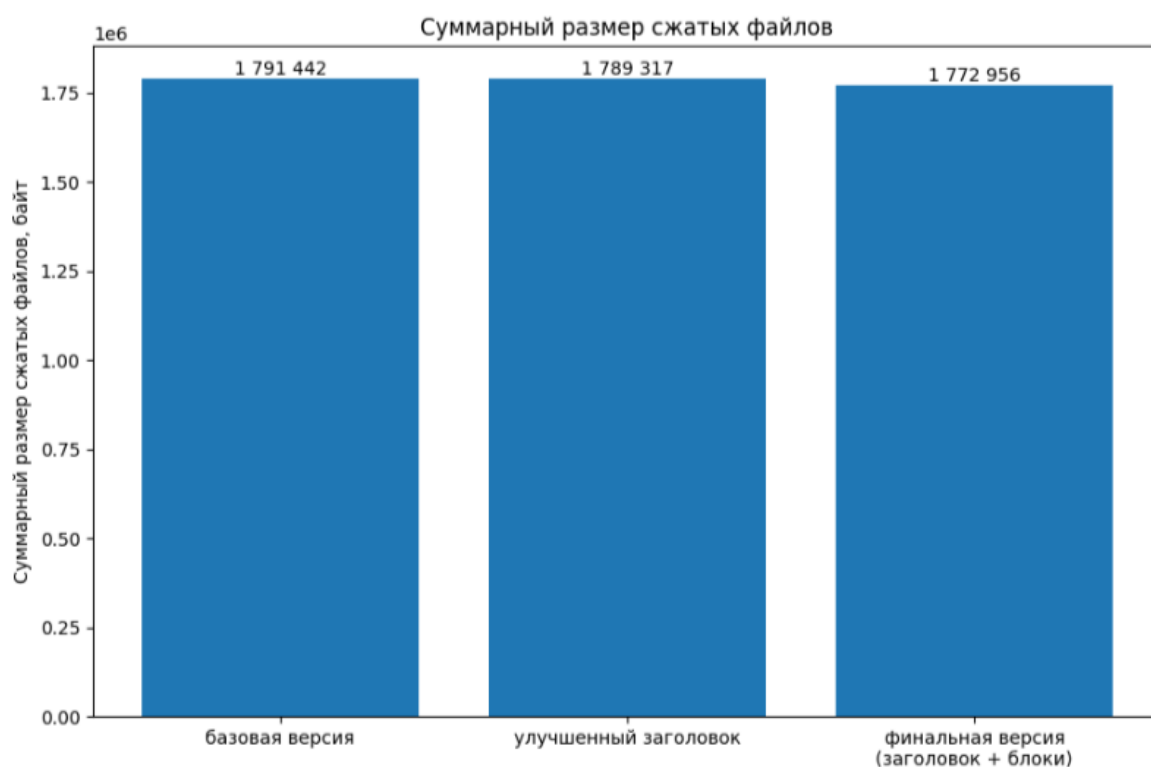
Рисунок 4 — График, показывающий суммарный размер сжатых файлов для трёх версий архиватора
