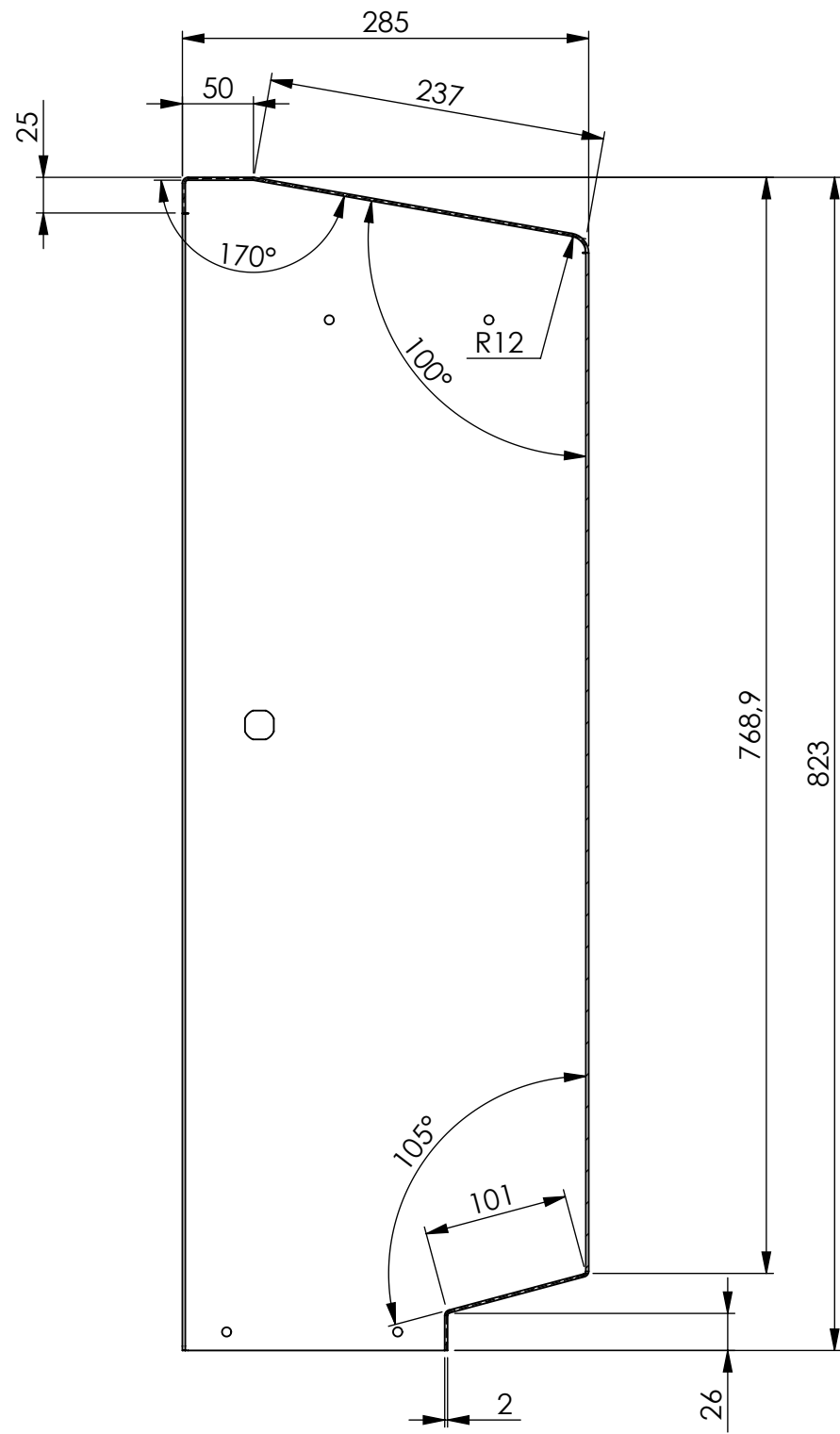
SECTION A-A
