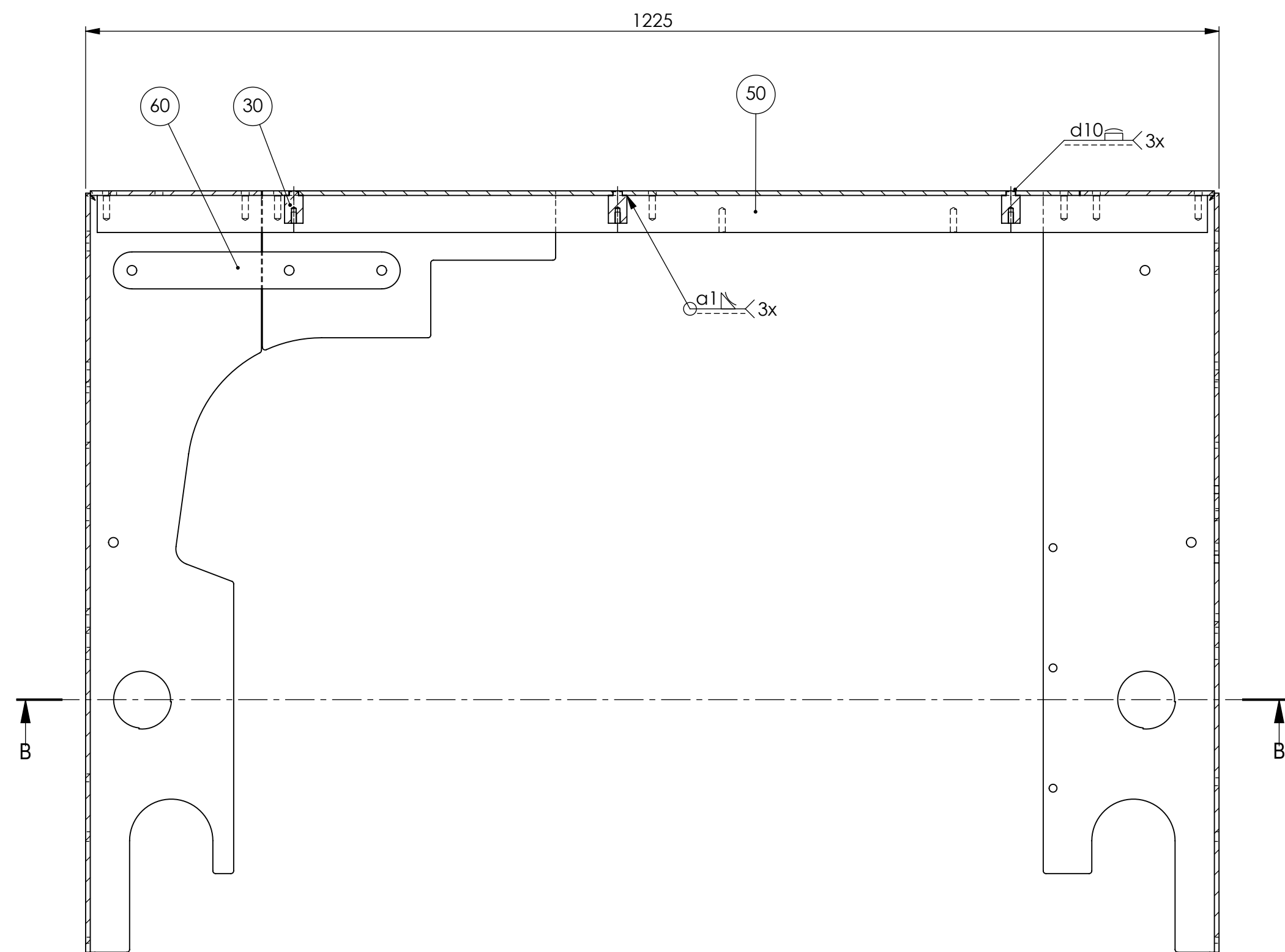
SECTION A-A
