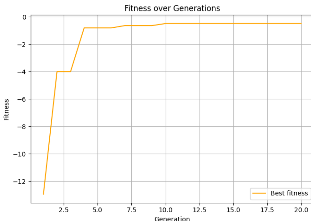
Slika 4: Vrednost funkcije prilagođenosti najbolje jedinice tokom 20 generacija kada se predviđa jedna nedostajuća vrednost
