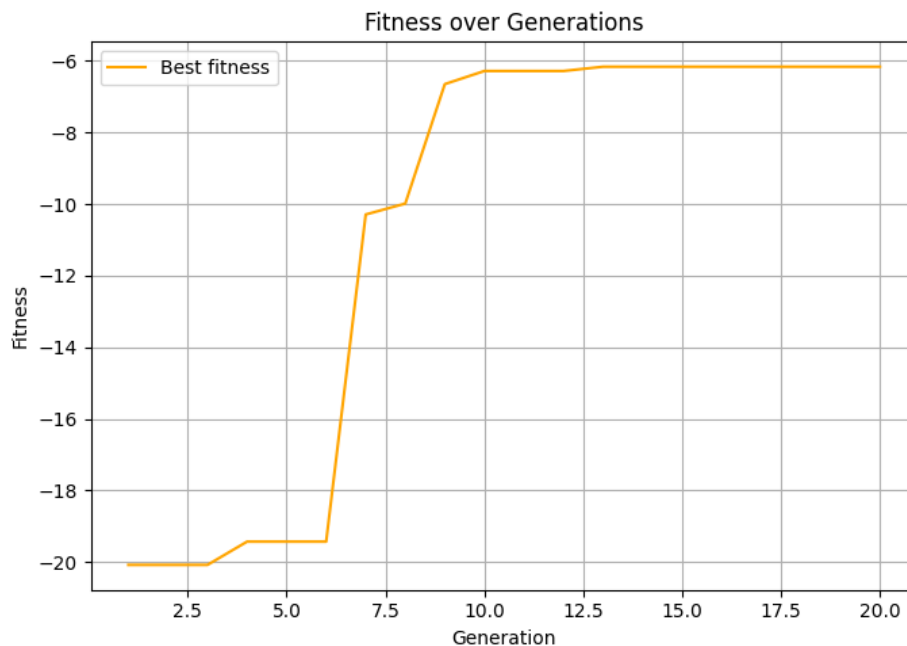
Slika 6: Vrednost funkcije prilagođenosti najbolje jedinke tokom 20 generacija u slučaju kada se predviđaju dve nedostajuće vrednosti
