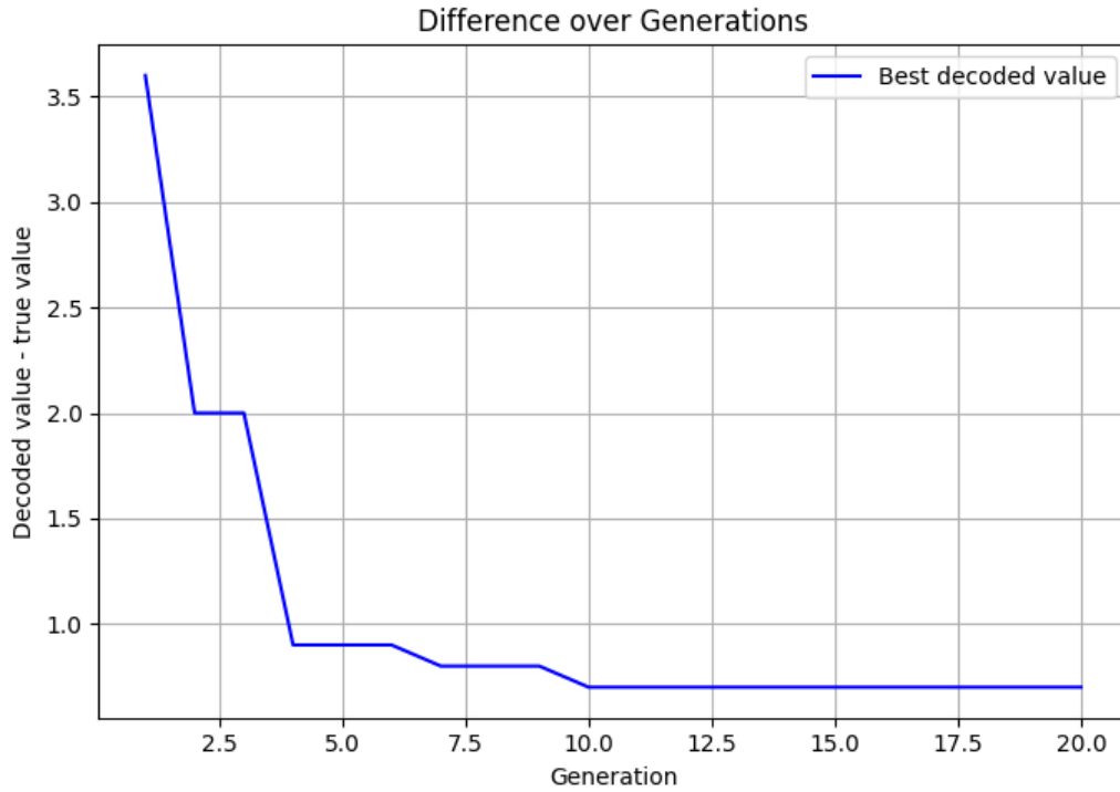
Slika 5: Apsolutna razlika između stvarne vrednosti i najbolje predviđene vrednosti kroz 20 generacija
