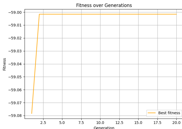
Slika 8: Vrednost funkcije prilagođenosti najbolje jedinice tokom 20 generacija u slučaju kada se predviđa jedna vrednost bez dostupne tačne vrednosti za poređenje
