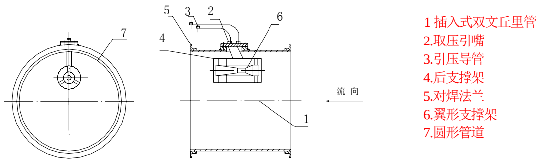
图 1 插入式双文丘里管插入圆形管道简图
