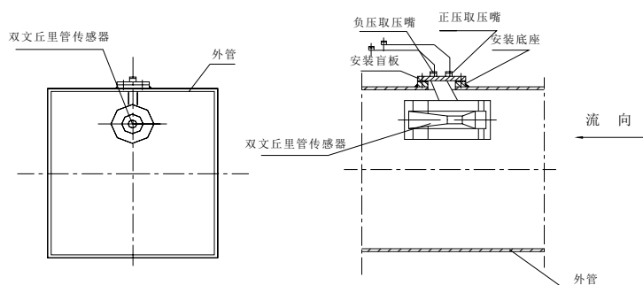
插入式双文丘里管矩形管道典型图例
