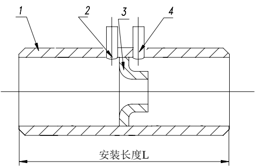
1. 外管 2. 正压取压嘴 3. 标准喷嘴 4. 负压取压嘴.
