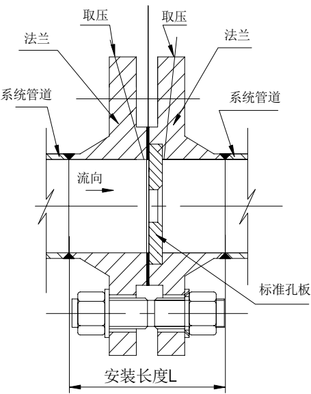
A 标准孔板图例
