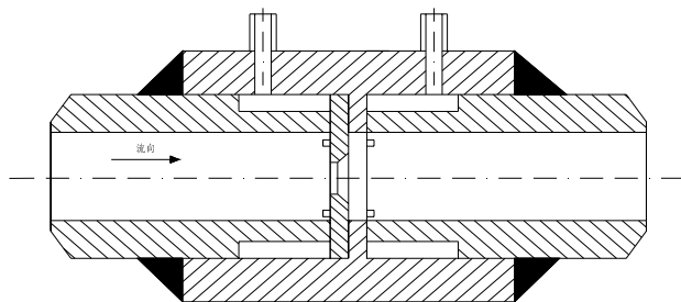
B 焊接及八槽孔板图例
