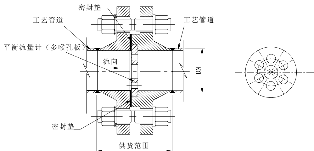
平衡流量计法兰夹持式图例
