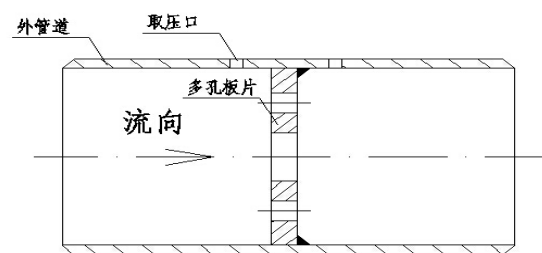
平衡流量计带外管对焊式图例
