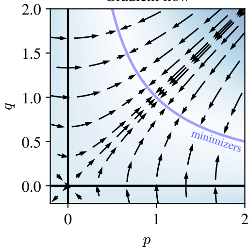
Gradient flow
