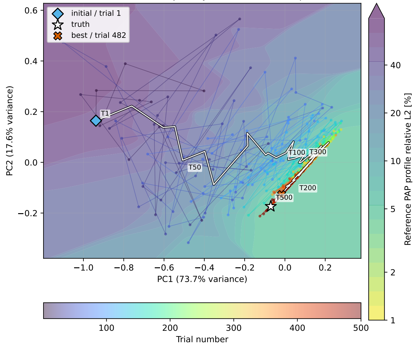
CMA-ES search trajectory in the fixed PCA space
