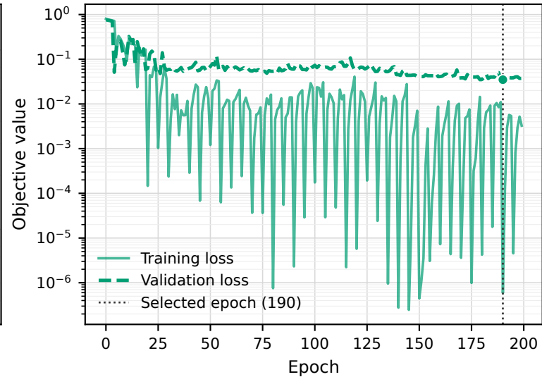
Global MLP
