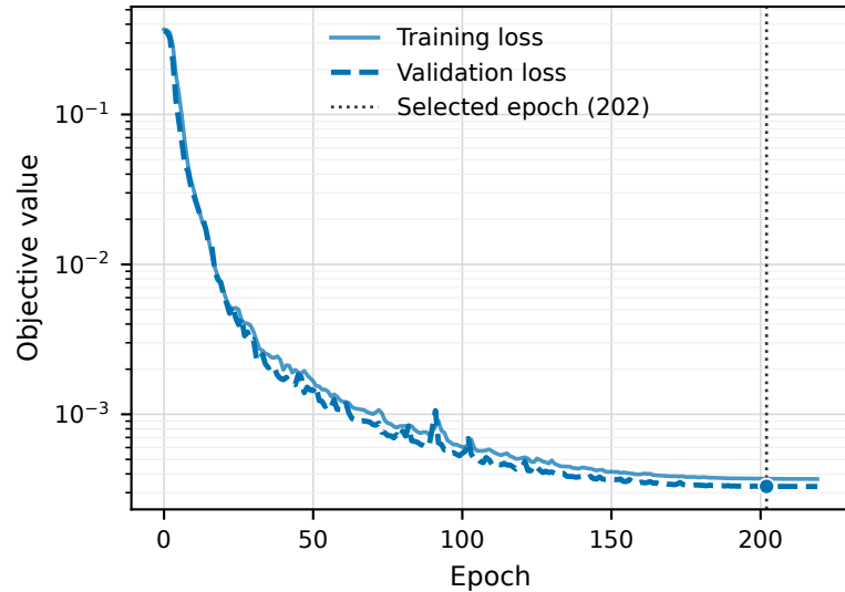
FFNO
