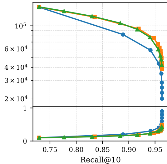
SIFT-500M
