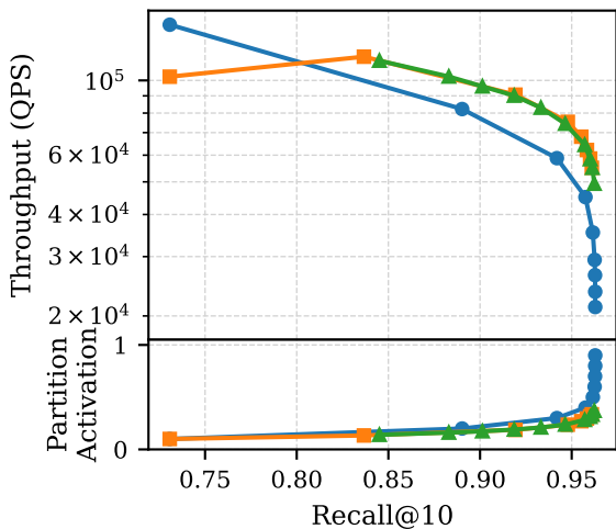
SIFT-500M
