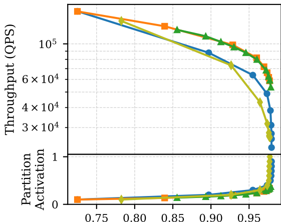
SIFT-500M
