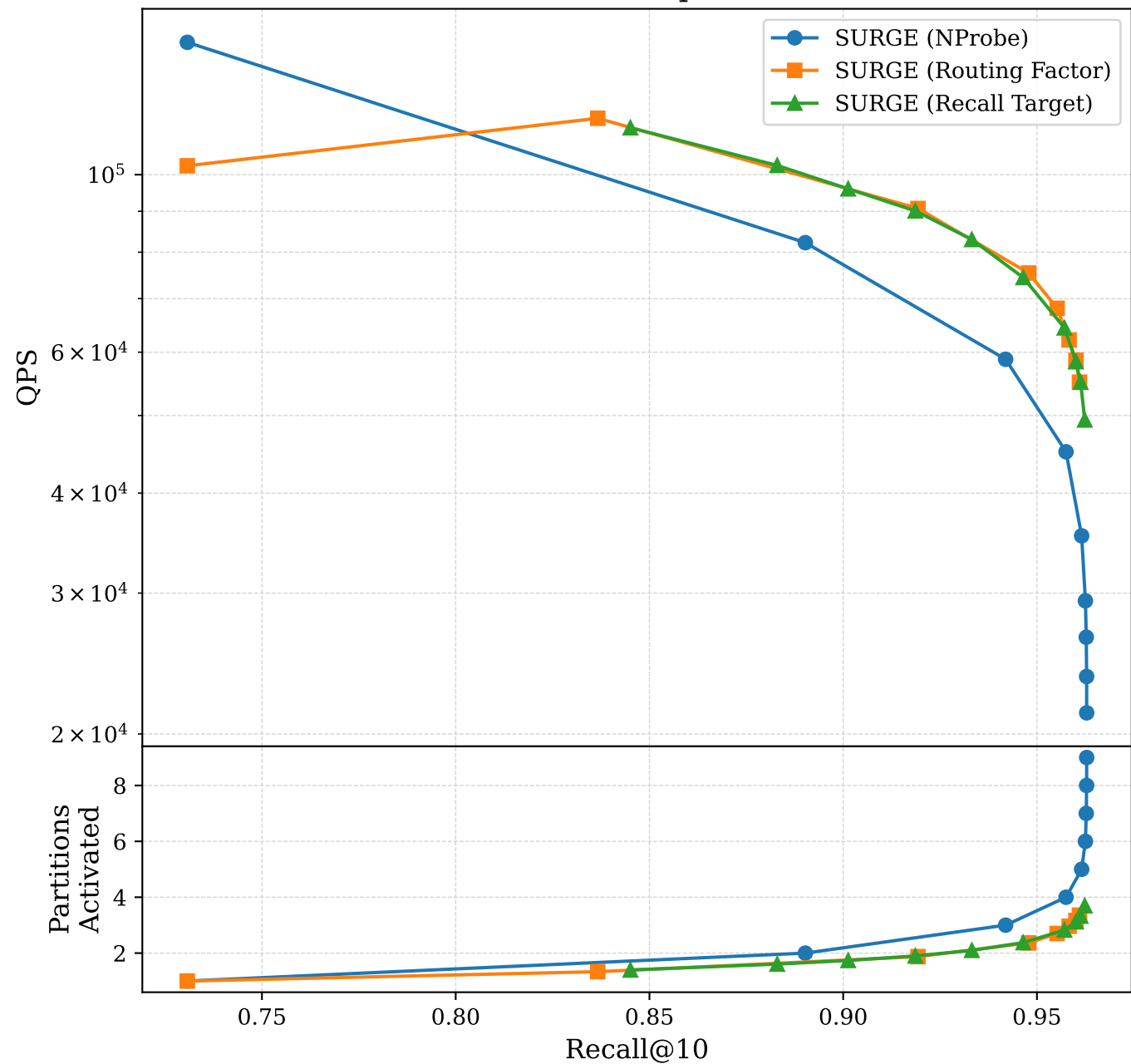
SIFT500M, 10 partitions
