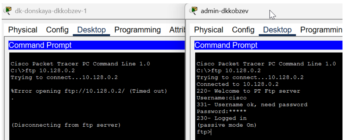
Рис. 2.3: Проверка доступа к web-серверу по протоколу FTP с устройства администратора
