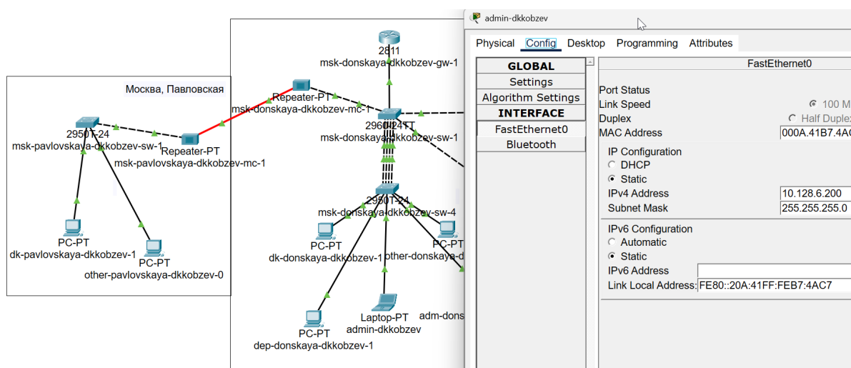
Рис. 2.1: Размещение ноутбука администратора в сети other-donskaya-1
