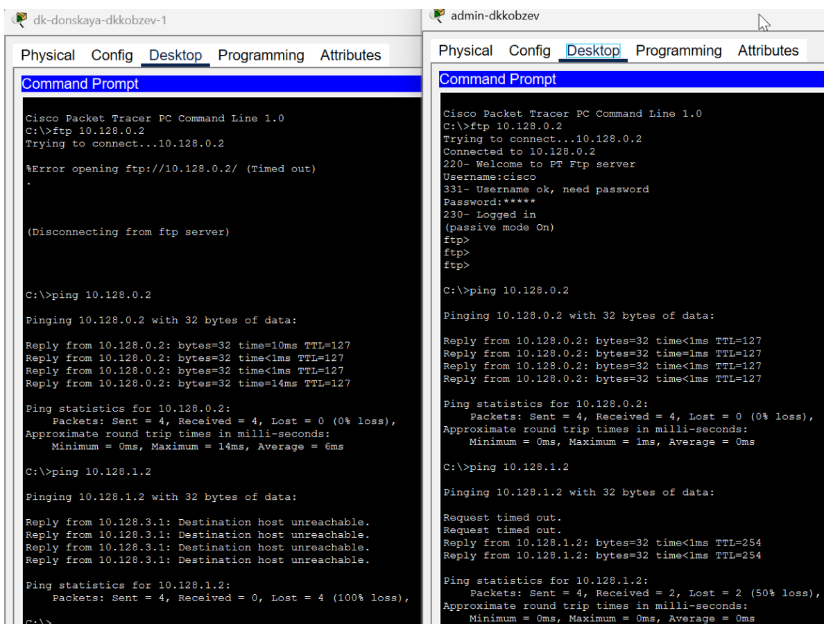
Рис. 2.7: Проверка корректности установленных правил доступа
