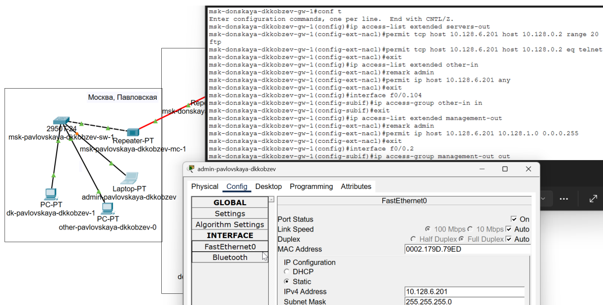
Рис. 2.8: Разрешения для администратора из сети Other на на Павловской
