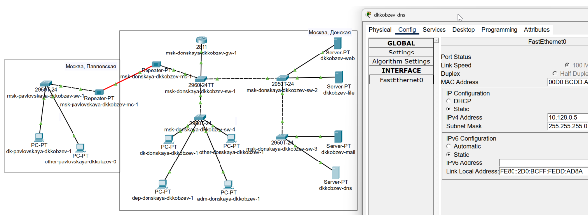
Рис. 2.1: Логическая схема локальной сети с добавленным DNS-сервером
