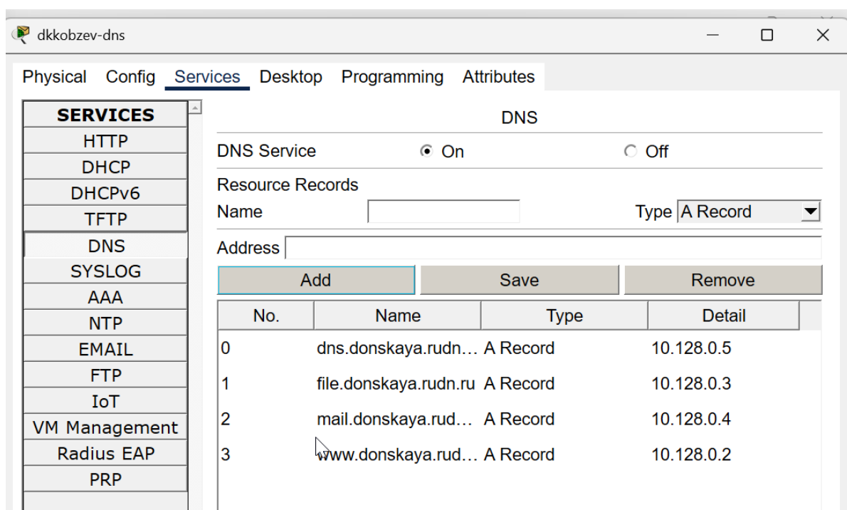
Рис. 2.2: Окно настройки сервиса DNS
