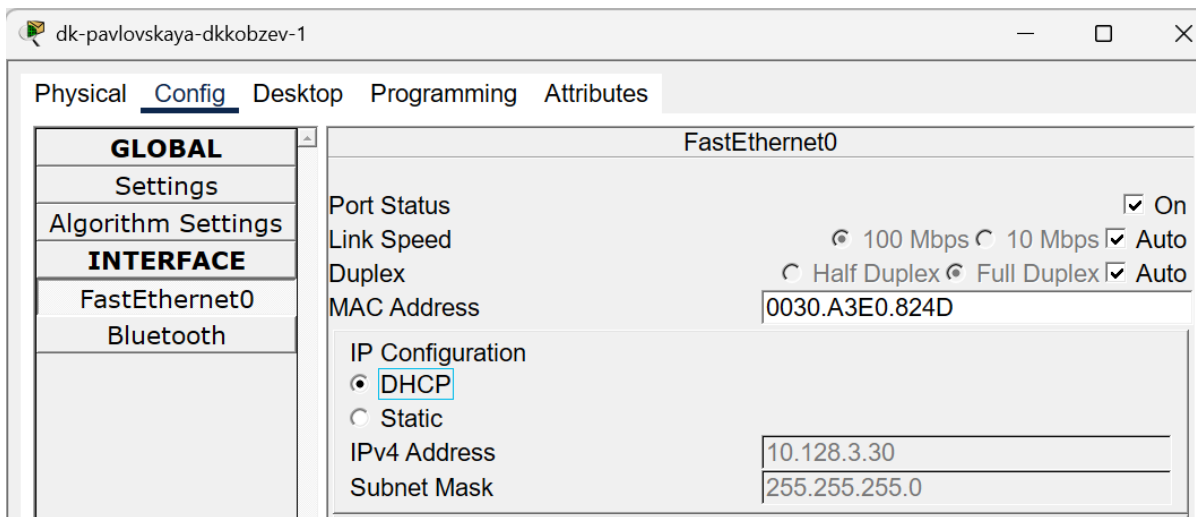
Рис. 2.5: Замена распределения адресов на оконечных устройствах
