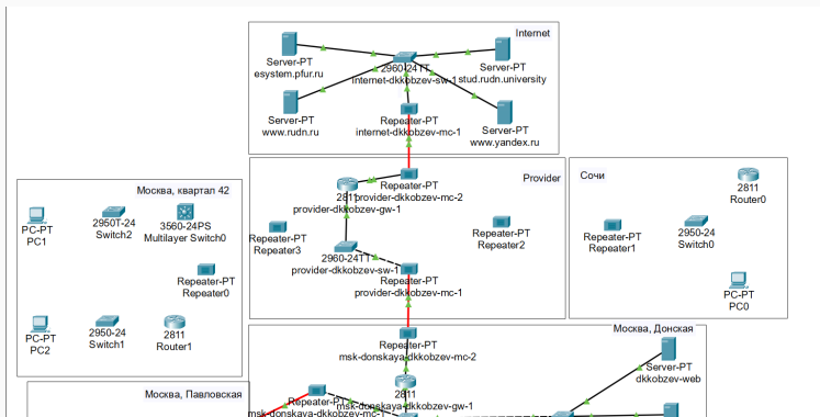
Рис. 1: Размещение необходимого оборудования на схеме
