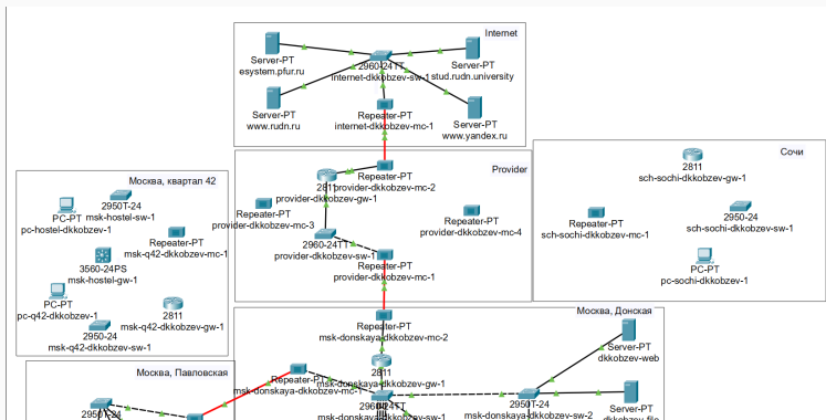
Рис. 2: Присваивание названий размещенным объектам
