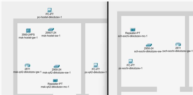
Рис. 7: Оборудование сети 42-го квартала и сети филиала
