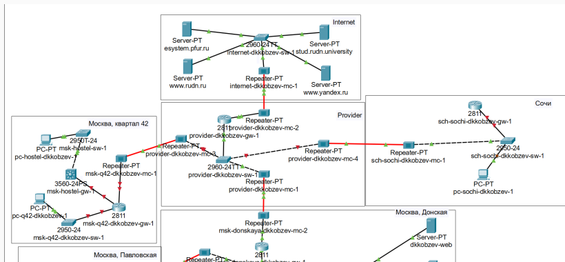
Рис. 8: Соединение объектов согласно схеме
