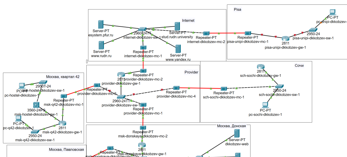
Рис. 2.1: Схема сети с дополнительными площадками
