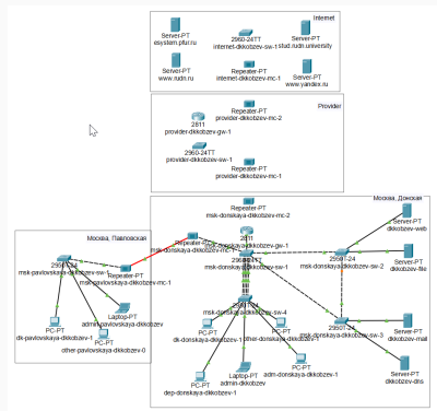
Рис. 1: Схема сети с выходом в Интернет
