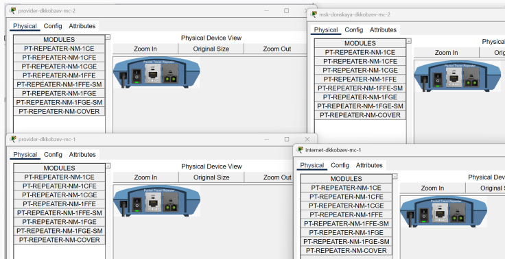
Рис. 5: Медиаконвертер с модулями PT-REPEATER-NM-1FFE и PT-REPEATER-NM-1CFE
