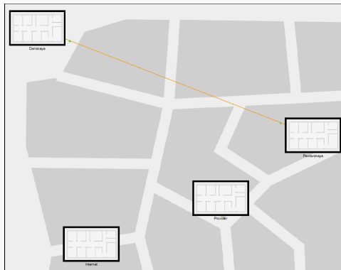
Рис. 2: Схема сети в физической рабочей области Packet Tracer
