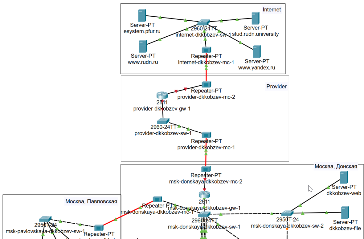
Рис. 2.6: Соединение объектов согласно схеме L1
