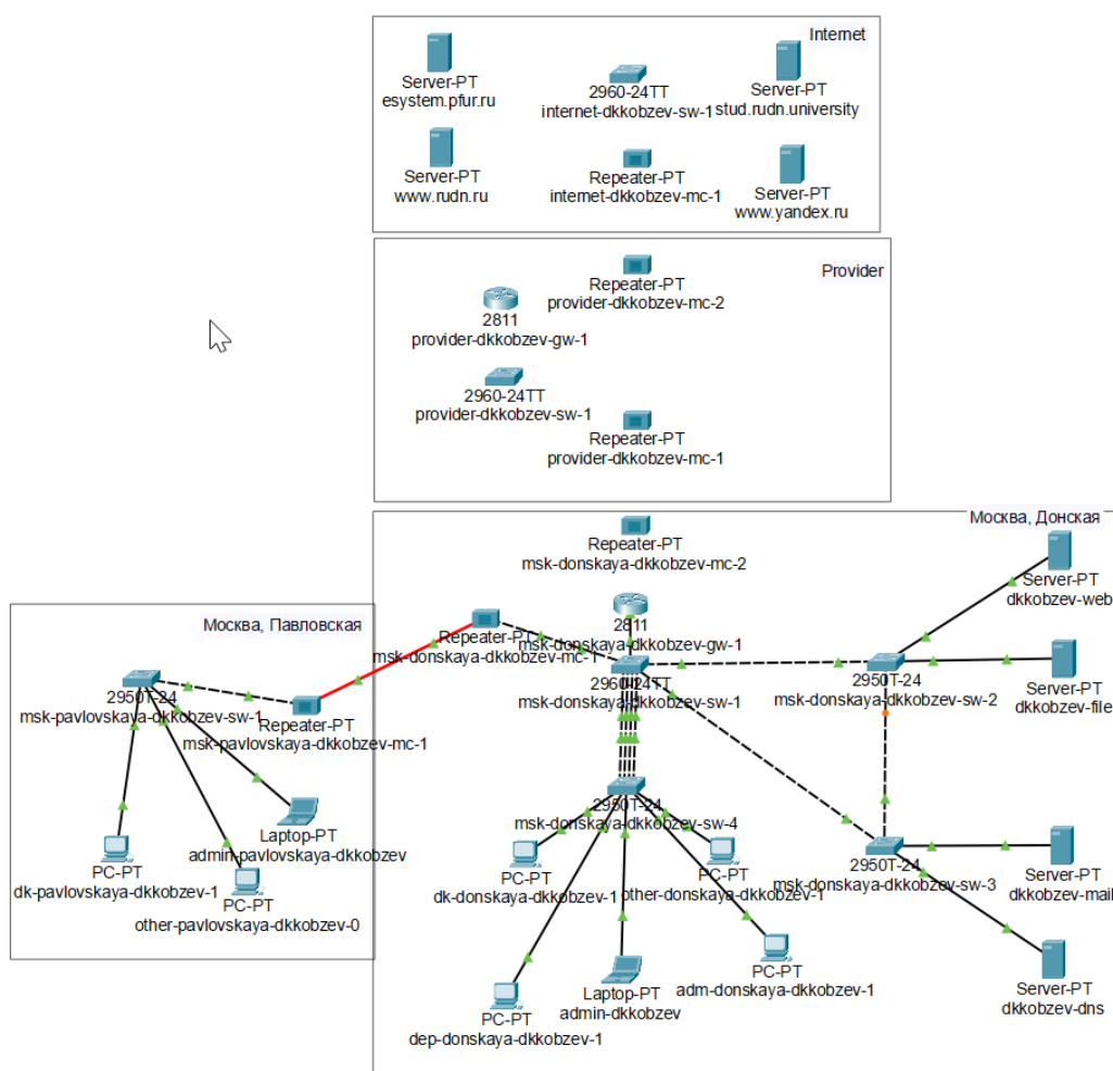
Рис. 2.1: Схема сети с выходом в Интернет
