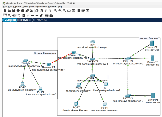
Рис. 12: Подключение повторителей
