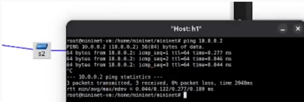
Рис. 14: Проверка связности
