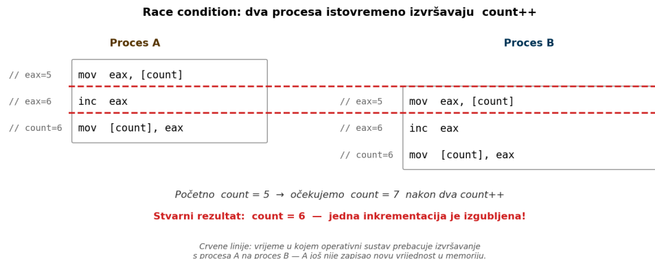
Slika 7.3: Stanje utrke ( race condition ) pri inkrementaciji dijeljenog brojača
