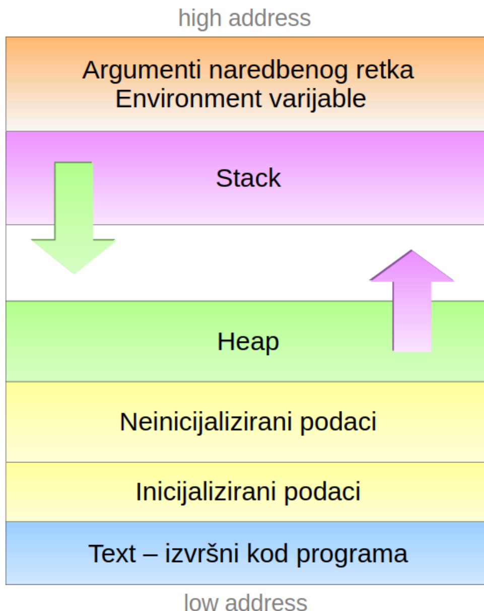
Slika 5.1: Memorijska slika UNIX procesa
