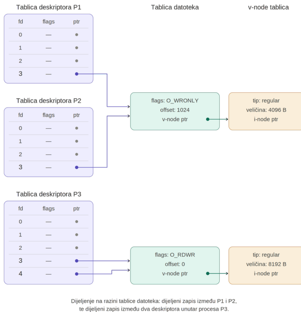
Slika 3.4: Dijeljenje na razini tablice datoteka
