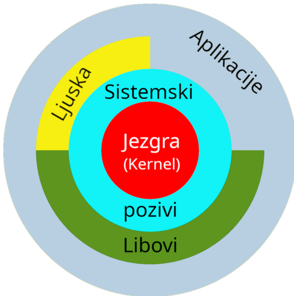
Slika 1.1: Arhitektura UNIX operacijskog sustava
