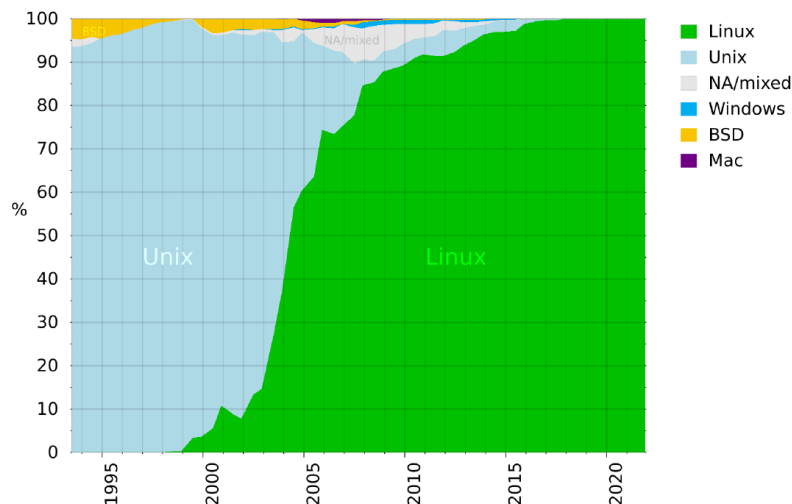
Slika 1.2: Operacijski sustavi na TOP500 superračunala
