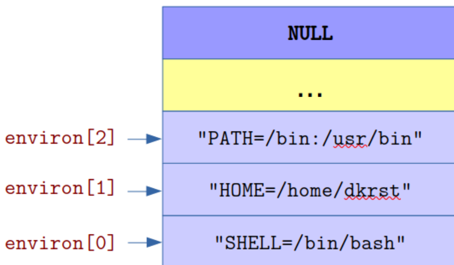
Slika 5.3: Organizacija varijabli okruženja u memoriji procesa
