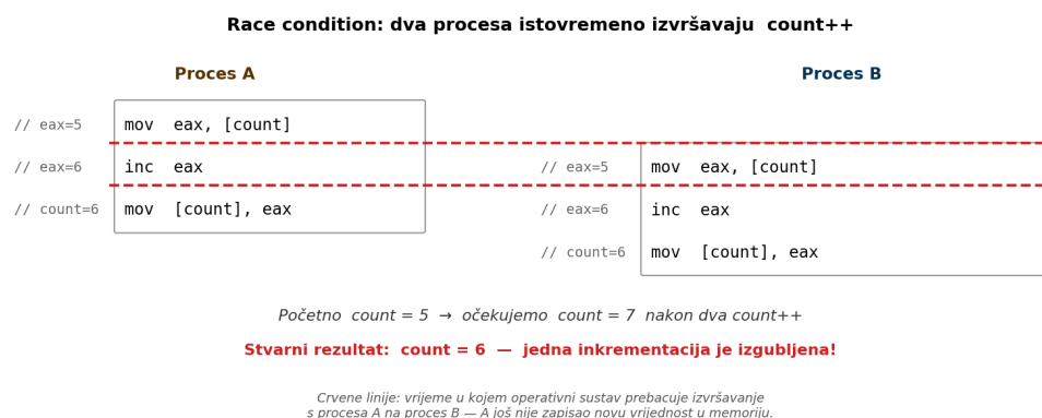
Slika 7.3: Race condition pri inkrementaciji dijeljenog brojača
