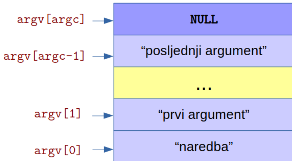
Slika 5.2: Organizacija argumenata naredbenog retka u memoriji procesa
