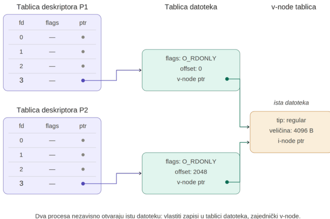
Slika 4.2: Dva procesa nezavisno otvaraju istu datoteku
