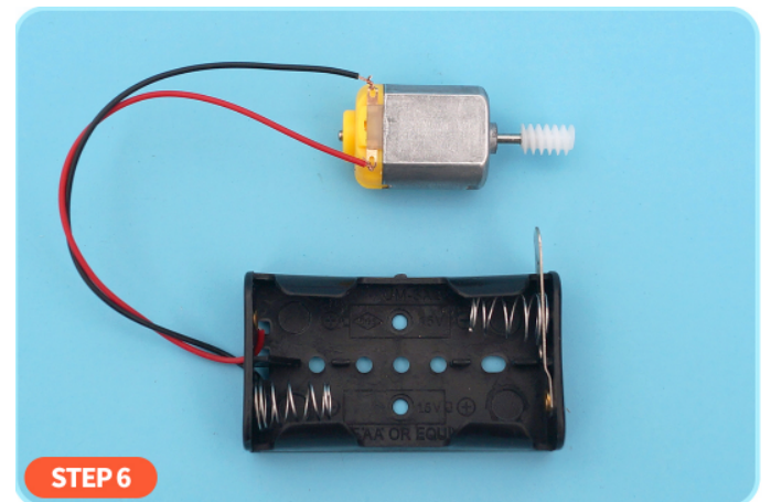
배터리 박스의 출력선을 모터에 연결합니다. 빨간선과 검은선의 위치를 그림과 동일하게 연결하세요. 금속 심선은 나선형으로 감아주세요. 금속 선을 모터 구리판 구멍에 넣고 3~4회 감아 고정합니다.
