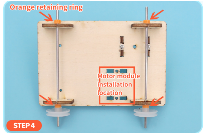
바퀴와 차축을 설치합니다. 흰색 폴리가 "모터 설치 위치" 방향을 향하도록 하고 돌출된 부분은 안쪽을 향하게 합니다.
