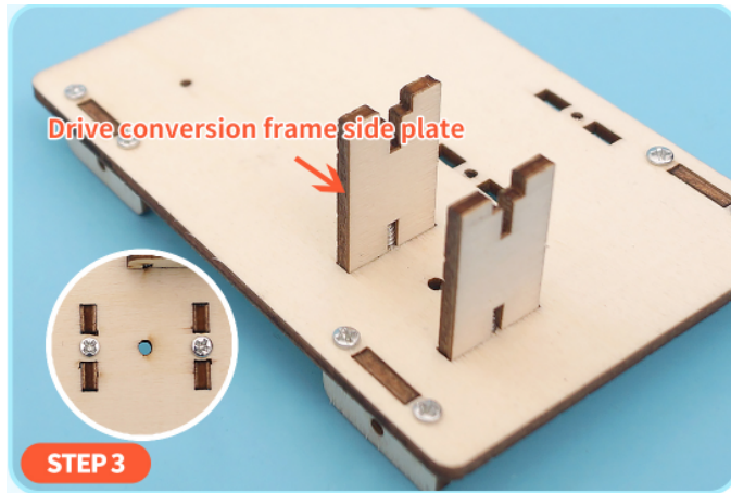
전달 변환 프레임의 측면 판을 메인 보드에 설치합니다. 7mm 나사를 사용해 아래쪽에서 고정합니다.
