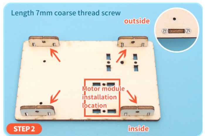
길이 7mm 나사를 사용하여 메인 보드에 4개의 차축 브라켓을 설치합니다. 모터 설치 위치 방향을 반드시 확인하세요.
