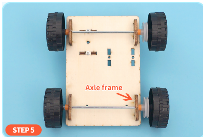
바퀴를 장착한 후 회전 저항을 확인합니다. 저항이 크다면 거리 조절 링과 차축 브라켓을 살짝 조정하세요.
