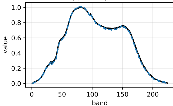
EM 4 | pred 1 | SAD 1.09°
