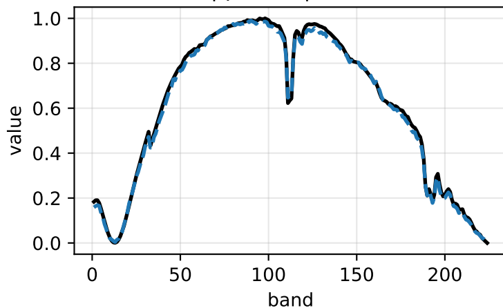
EM 3 | pred 2 | SAD 0.93°
