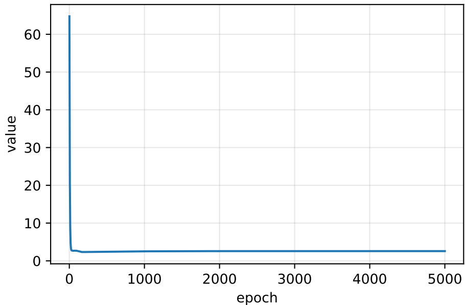
KL divergence
