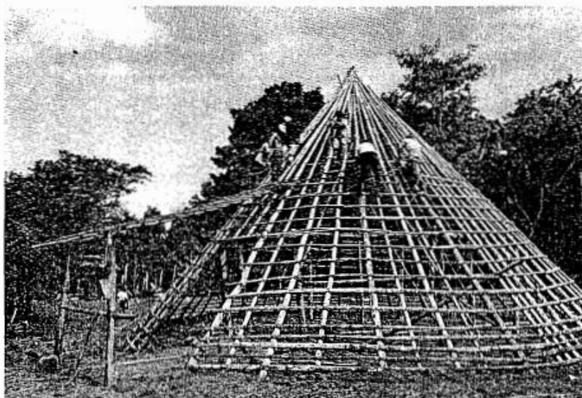
Construcción de ù sulè 'casa cónica tradicional' Kachàbali, Talamanca
