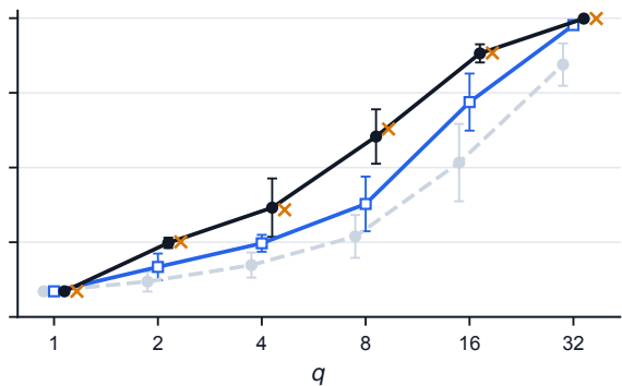
(d) Cycle-span 2-cells
