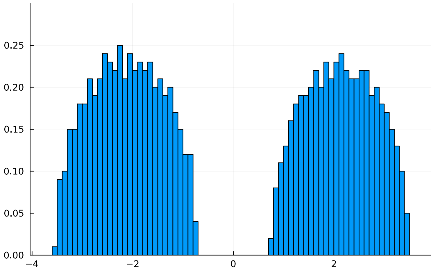
Eigenvalues of A_n + D_n
