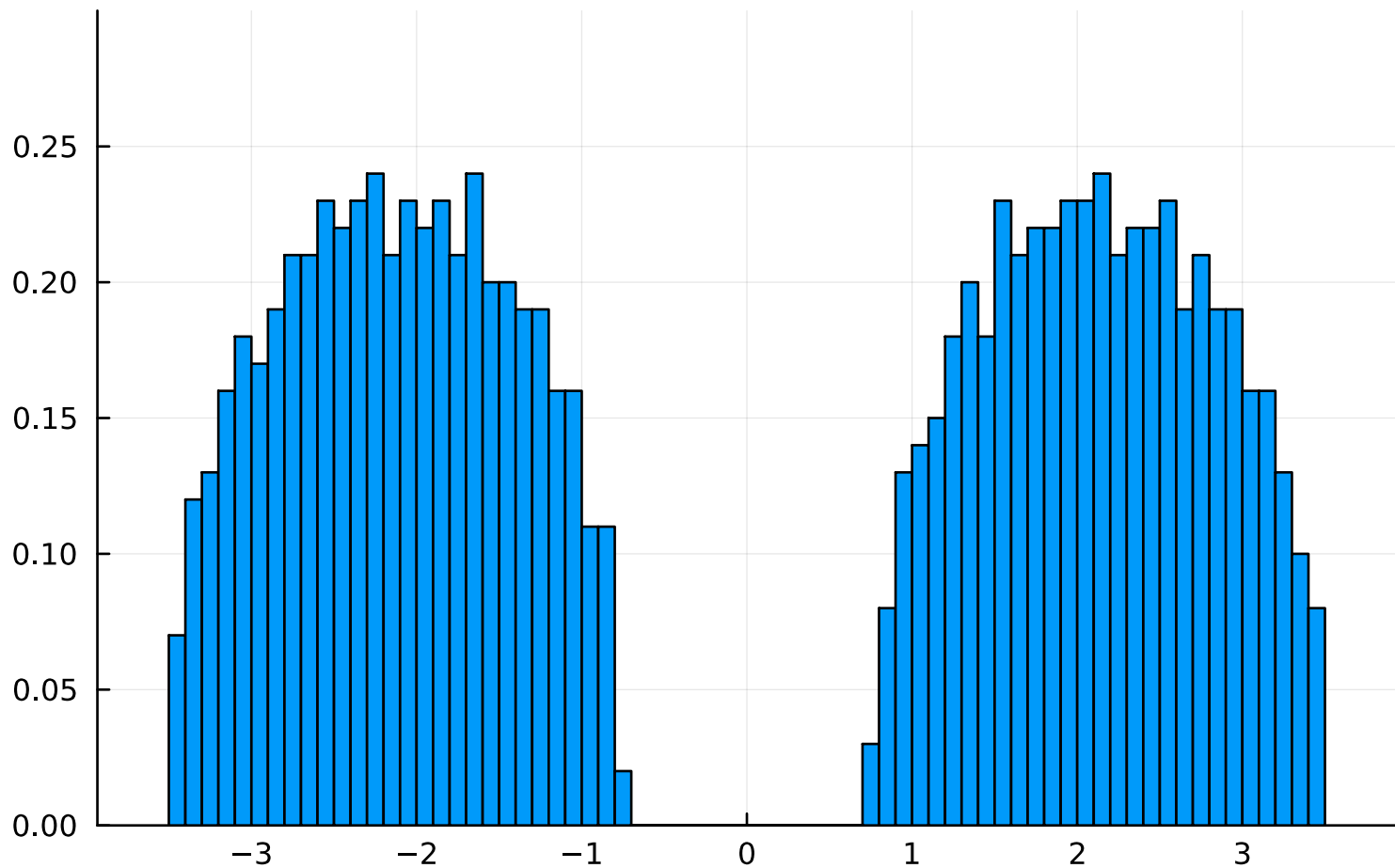
Eigenvalues of A_n + B_n
