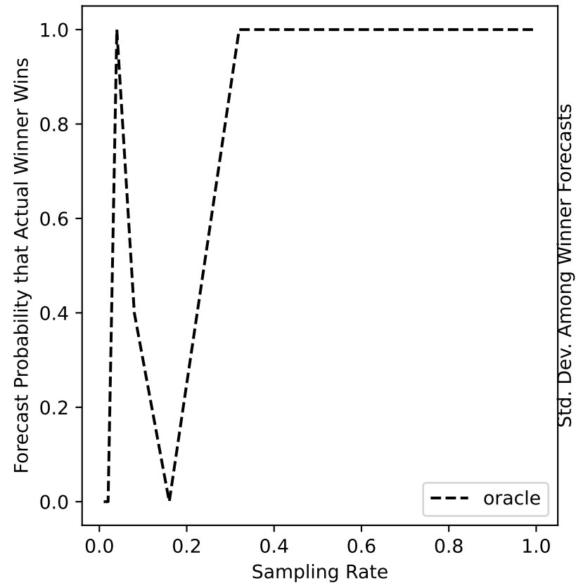
ers-17 Forecast
