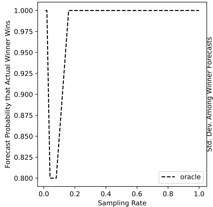
ers-23 Forecast
