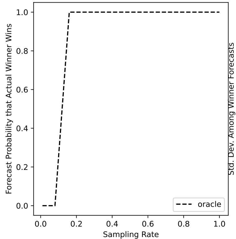
ers-30 Forecast
