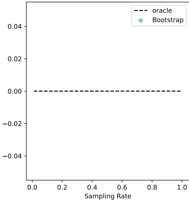
ers-30 Uncertainty
