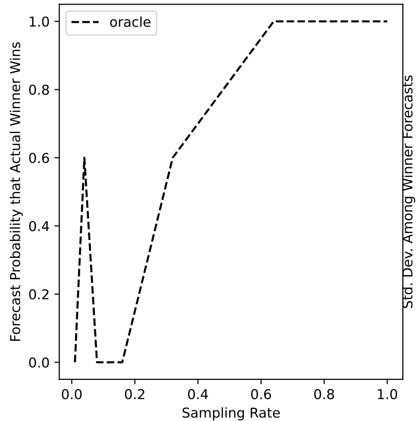
ers-47 Forecast
