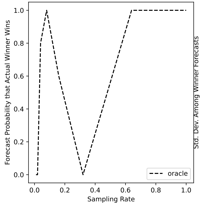
ers-49 Forecast
