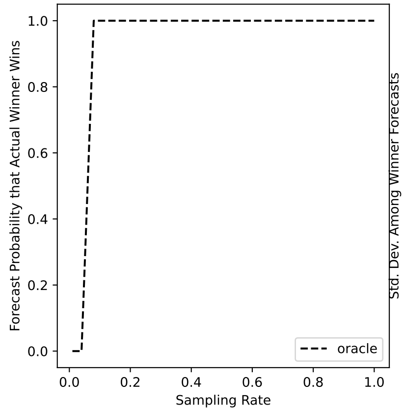
ers-53 Forecast
