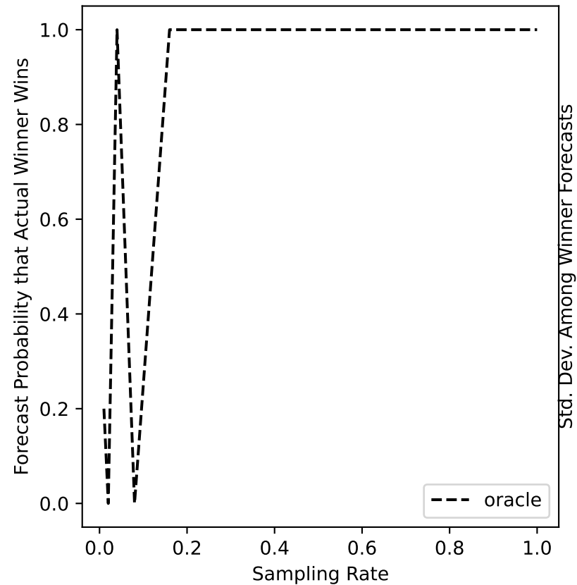
ers-60 Forecast
