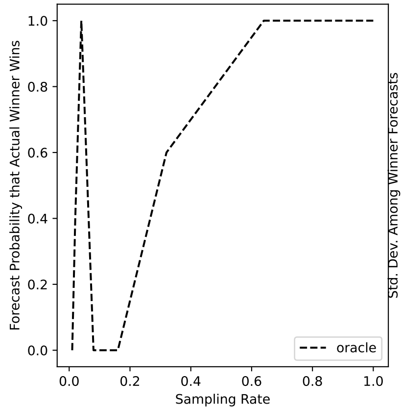
ers-62 Forecast
