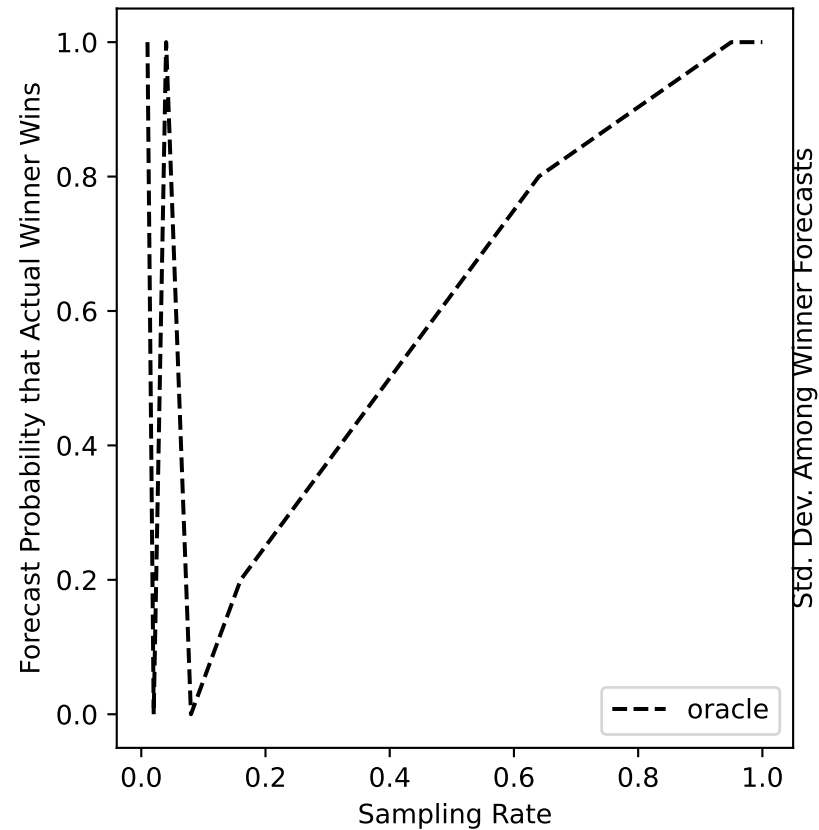
ers-73 Forecast
