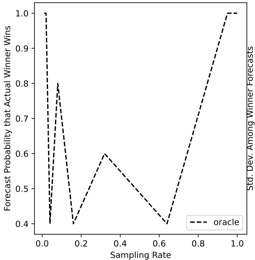
ers-81 Forecast
